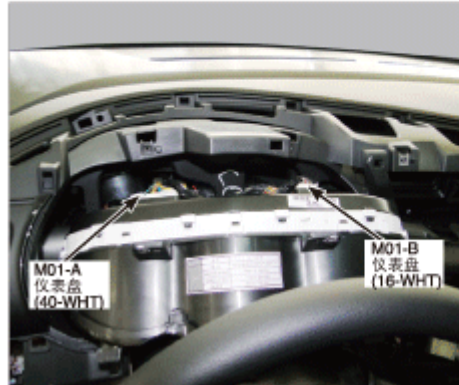
43.仪表板左侧
