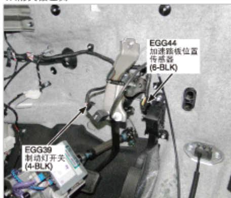
47.防火板左侧
