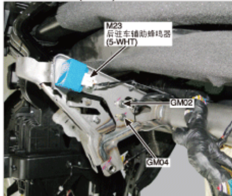
44.暖风总成左侧(后视图)
