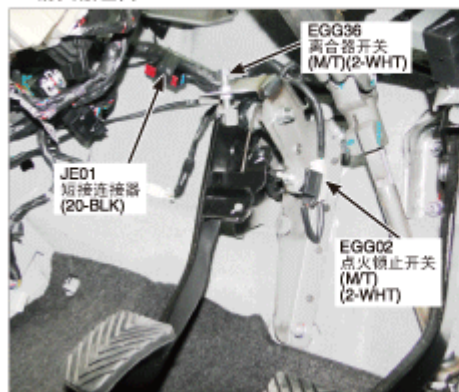
46.防火板左侧
