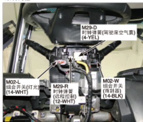
48.转向柱
