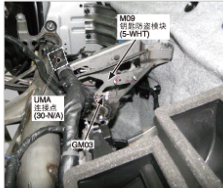
45.仪表板上部左侧
